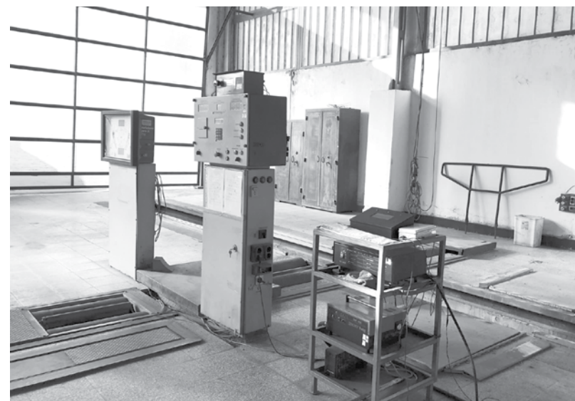
Диммер, газанализатор, спирална система - част от апаратурата, с която се правят замерванията по време на ГТП ФОТО: МОНИКА ИЛИЕВА
