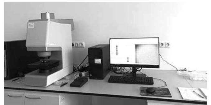
В Лабораторията по мониторинг на води се намира единственият в България микроскоп с инфрачервена спектроскопия LUMOS II на Bruker за анализ на микропластмаса ФОТО: УНИВЕРСИТЕТ „ПРОФ. Д-Р АСЕН ЗЛАТАРОВ“
